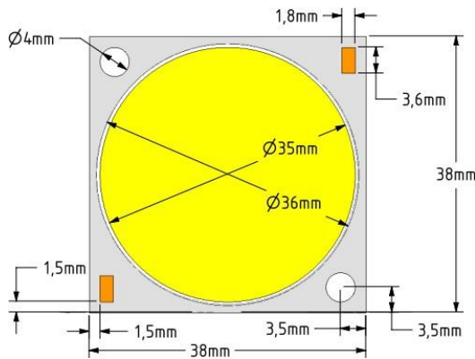
Üst Görünüş
